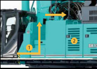
1 Ajout d'une passerelle côté gauche Des marches et rambardes de sécurité sur le réservoir d'huile hydraulique facilitent l'accès à la tourelle.
