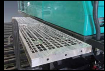
Passerelles amovibles Des passerelles sont prévues sur les côtés gauche et droit de la tourelle, pour sécuriser l'accès à l'entretien.
